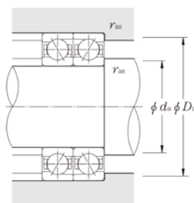
Парная установка по схеме «Х»
