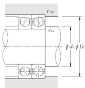
Парная установка по схеме «О»
