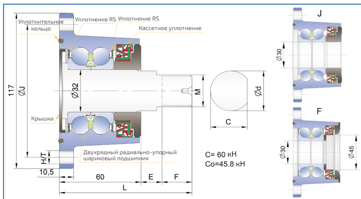
Чертеж подшипникового узла IL-50
