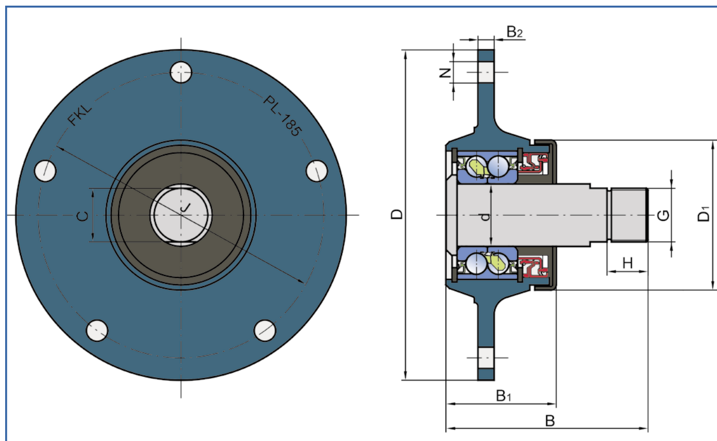
Подшипник дисковой бороны
