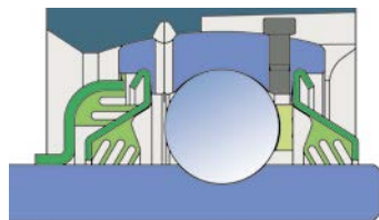
Рис. 10 Уплотнение TDT
